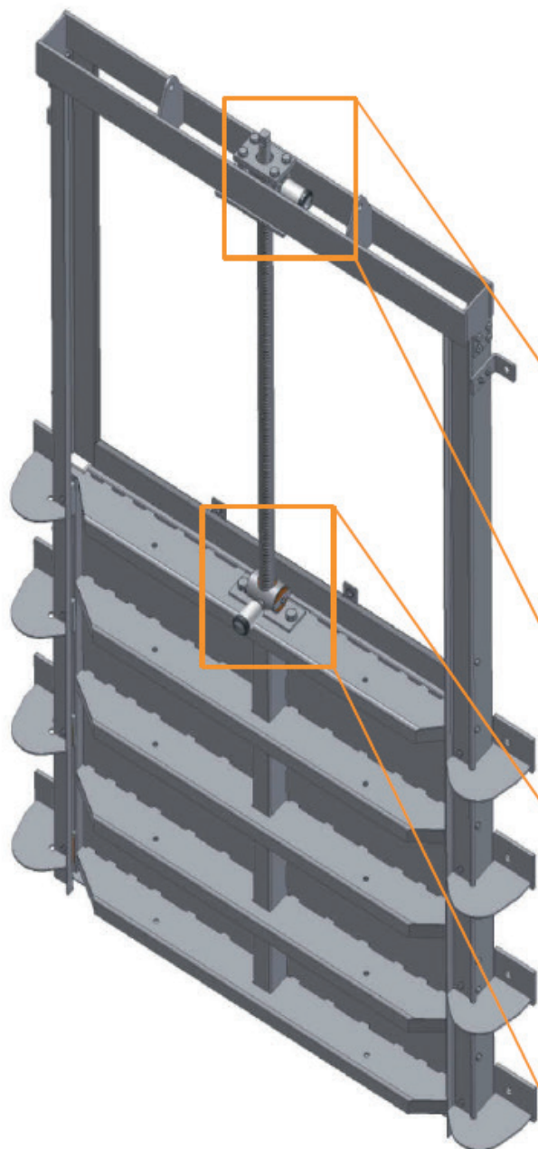
XL4 1600 x 1600 ze zdecentralizowanym systemem smarowania łożyska i nakrętki wrzeciona
