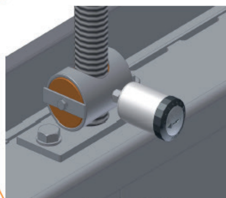
Smarowniczka zainstalowana na nakrętce wrzeciona
