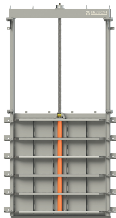
Zasuwa XL4 2100x2100 z półokrągłym dnem z napędem elektrycznym
