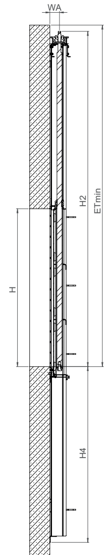
XL4 z płytą opuszczaną 1500 x 1500 mm widok z boku
